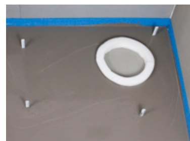
Nivåmarkörer för exakta höjder.
