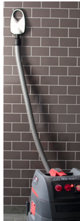
Suger sig fast mot underlaget vid anslutning till dammsugare.
